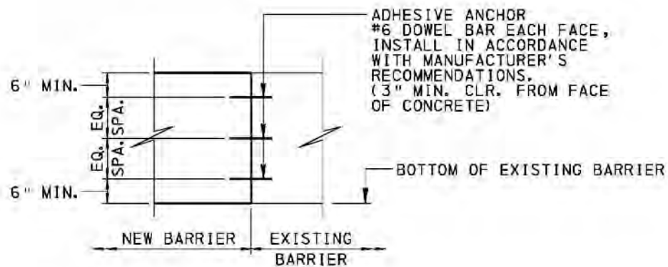
ELEVATION B-B
